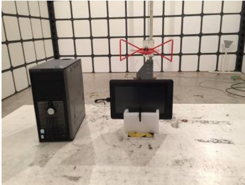
30MHz~1000MHz
