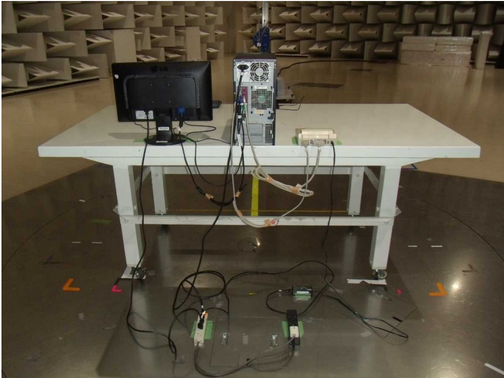
Setting(Rear)
