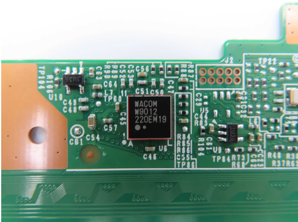
EMR Module
