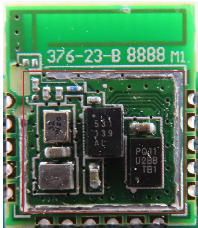
BT Module
