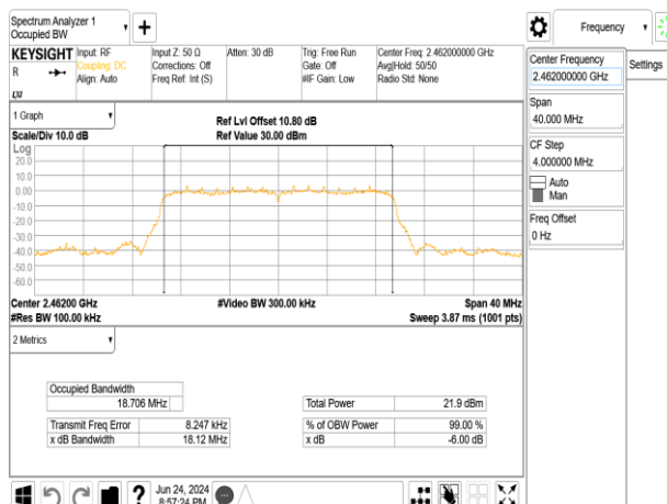
802.11ax_20MHz_Chain0_2462MHz
