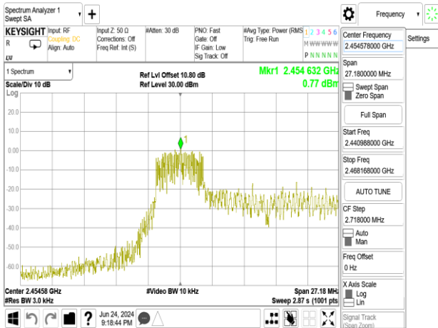
802.11ax_20MHz_Chain0_2462MHz_RU52_40
