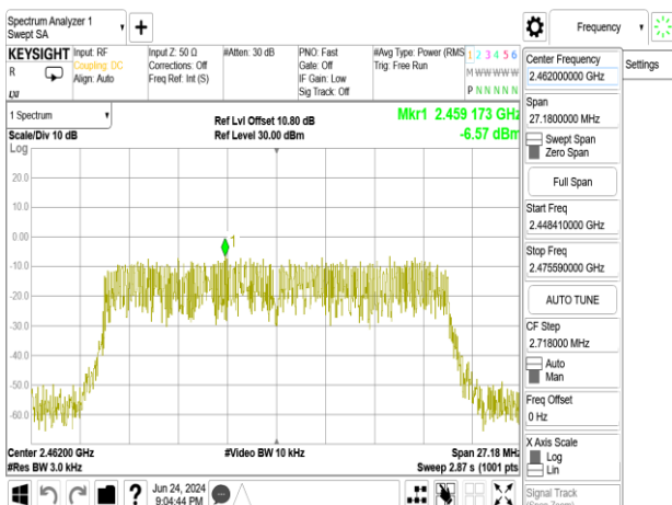
802.11ax_20MHz_Chain0_2462MHz_SU
