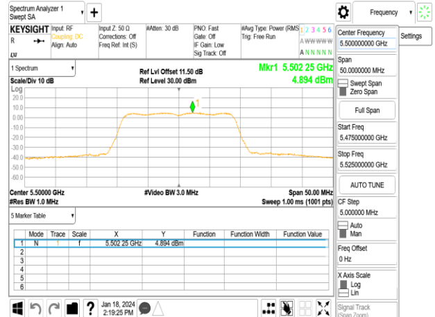
802.11n_20MHz_Chain0_5500MHz
