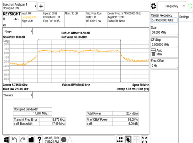
802.11n_20MHz_Chain0_5745MHz
