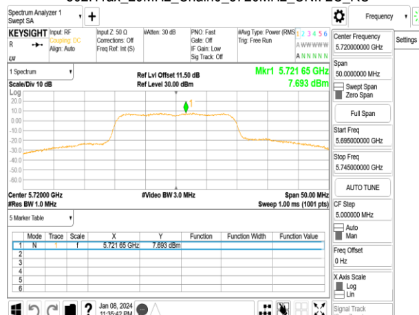
802.11ax_20MHz_Chain0_5720MHz_UNII 2C_SU
