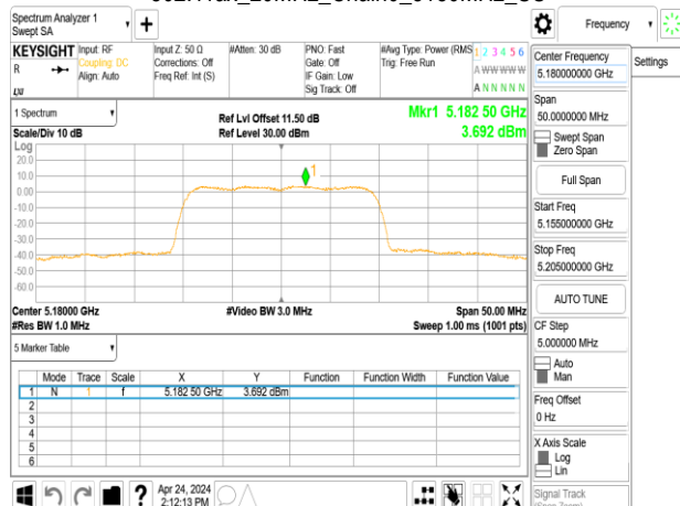
802.11ax_20MHz_Chain0_5180MHz_SU
