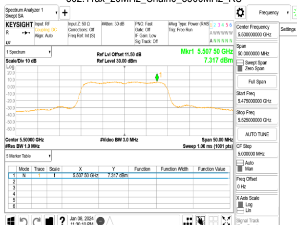
802.11ax_20MHz_Chain0_5500MHz_RU106_53
