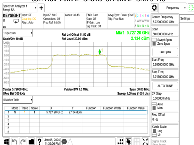
802.11ax_20MHz_Chain0_5720MHz_UNII 3 SU
