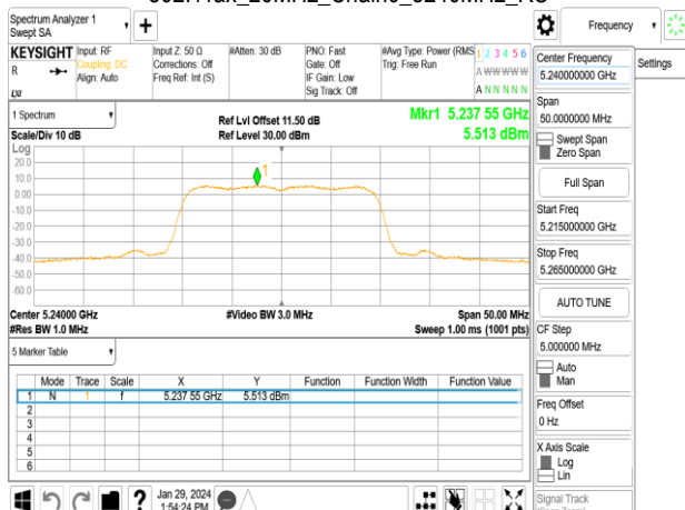
802.11ax_20MHz_Chain0_5240MHz_RU
