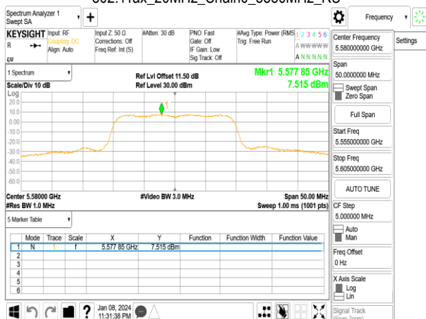
802.11ax_20MHz_Chain0_5580MHz_SU
