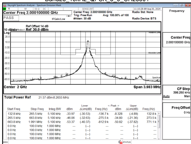
Band23_15kHz_QPSK_3_9_CH25600
