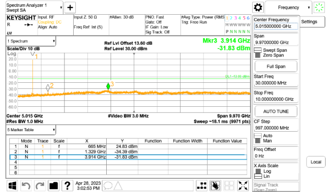
Cat-M1 Band71_20MHz_QPSK_RB1_0_CH133297
