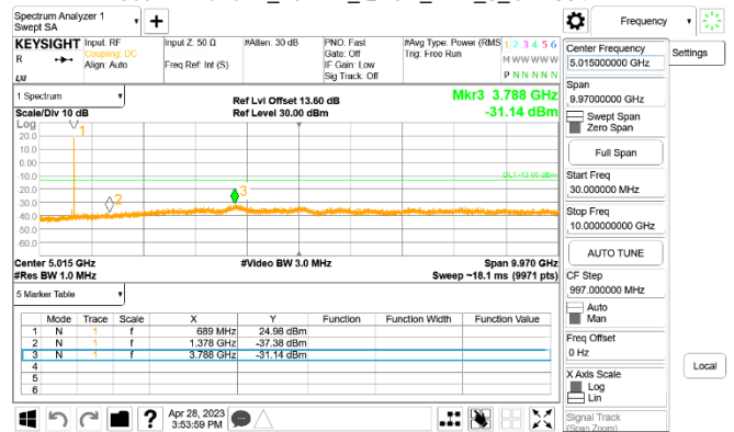
Cat-M1 Band71_10MHz_QPSK_RB1_0_CH133442
