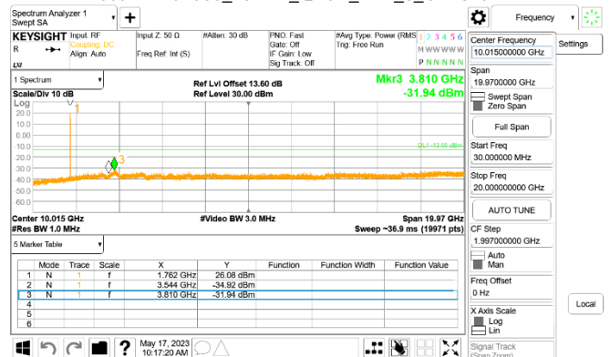
Cat-M1 Band66_20MHz_QPSK_RB1_0_CH132572
