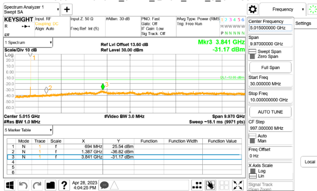
Cat-M1 Band71_5MHz_QPSK_RB1_0_CH133447
