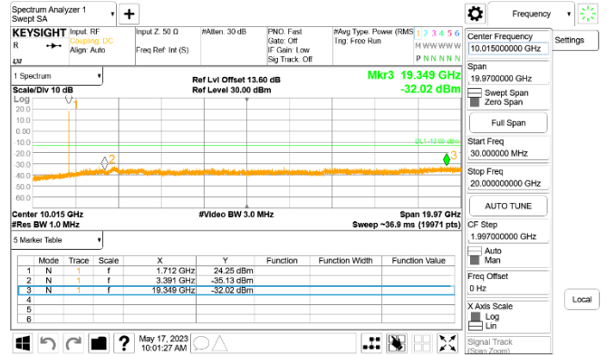
Cat-M1 Band66_20MHz_QPSK_RB1_0_CH132322
