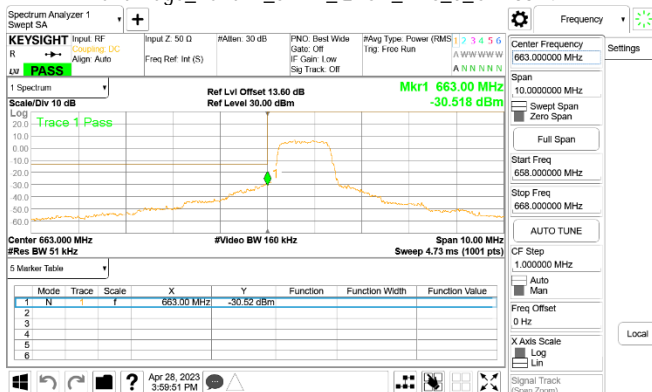
Band Edge_Band71_5MHz_QPSK_RB6_0_CH133147
