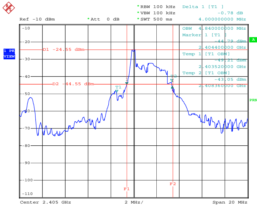
20 dB/99% Bandwidth Plot on 錯誤! 找不到參照來源。
