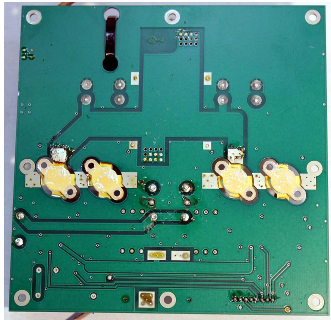
PAM-606 (PA module) bottom
