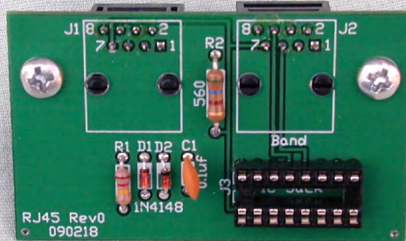
RJ45 top
