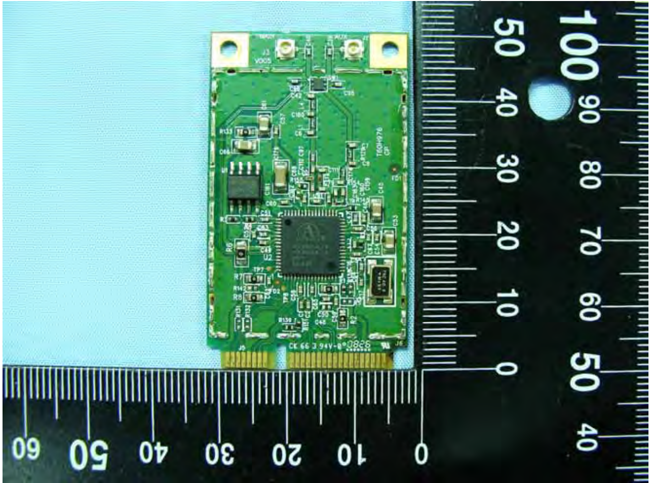
WLAN Module
