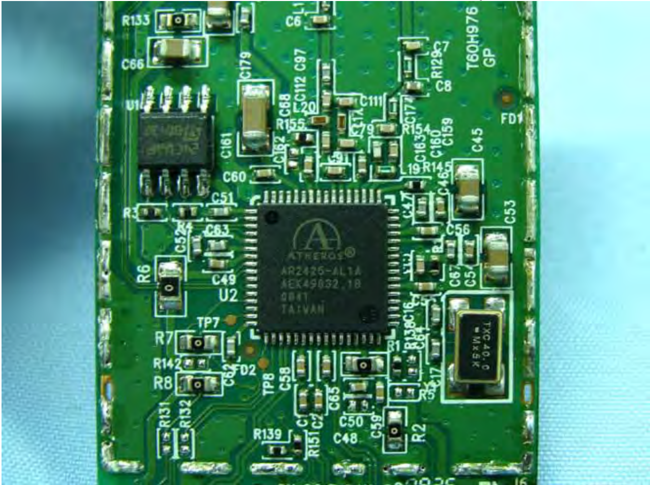
WLAN Module
