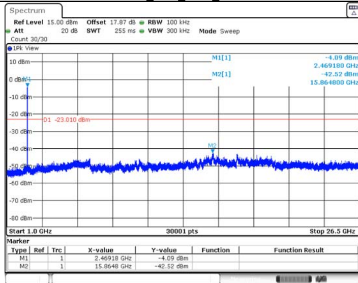
11N20MIMO_Ant2_2462_1000~26500
