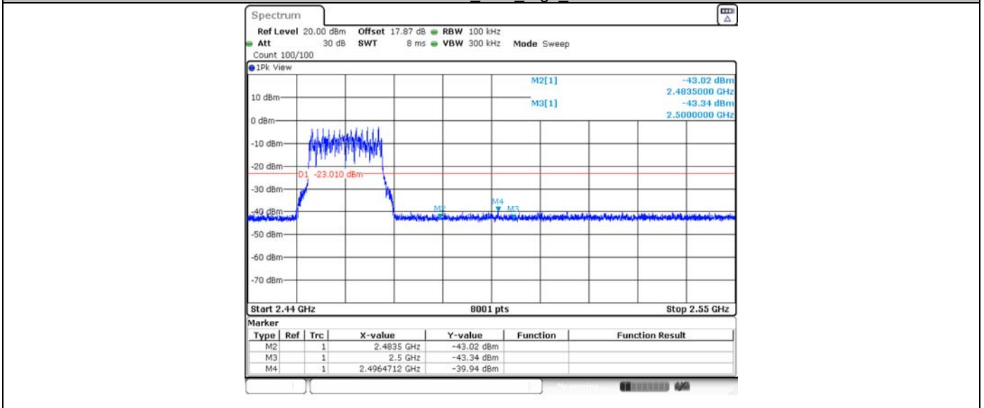
11N20MIMO_Ant2_High_2462
