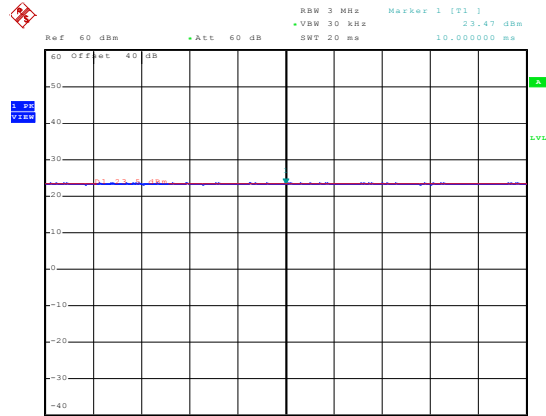
1880MHz - CW
