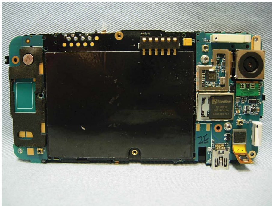
(20) EUT Photo
