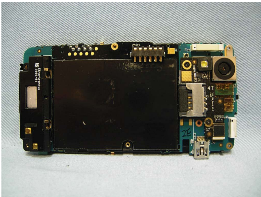
(18) EUT Photo
