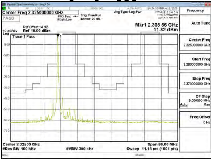
Band30_10MHz_QPSK_1_49_CH27710
