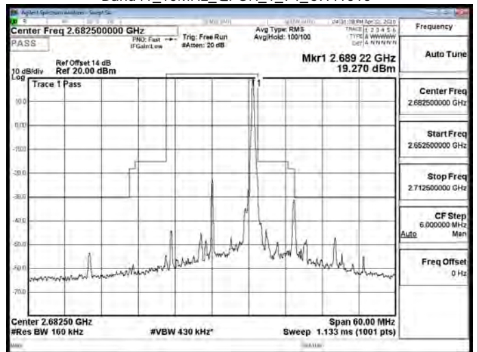
Band41_15MHz_QPSK_1_74_CH41515
