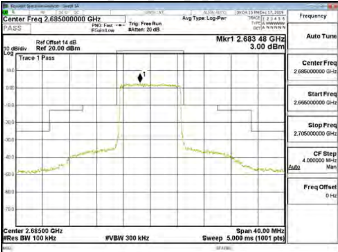
Band41_10MHz_QPSK_50_0_CH41540
