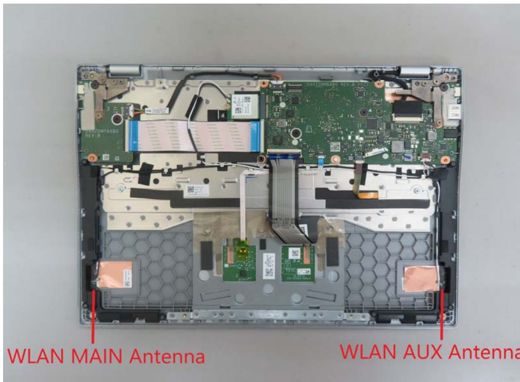
Antenna
