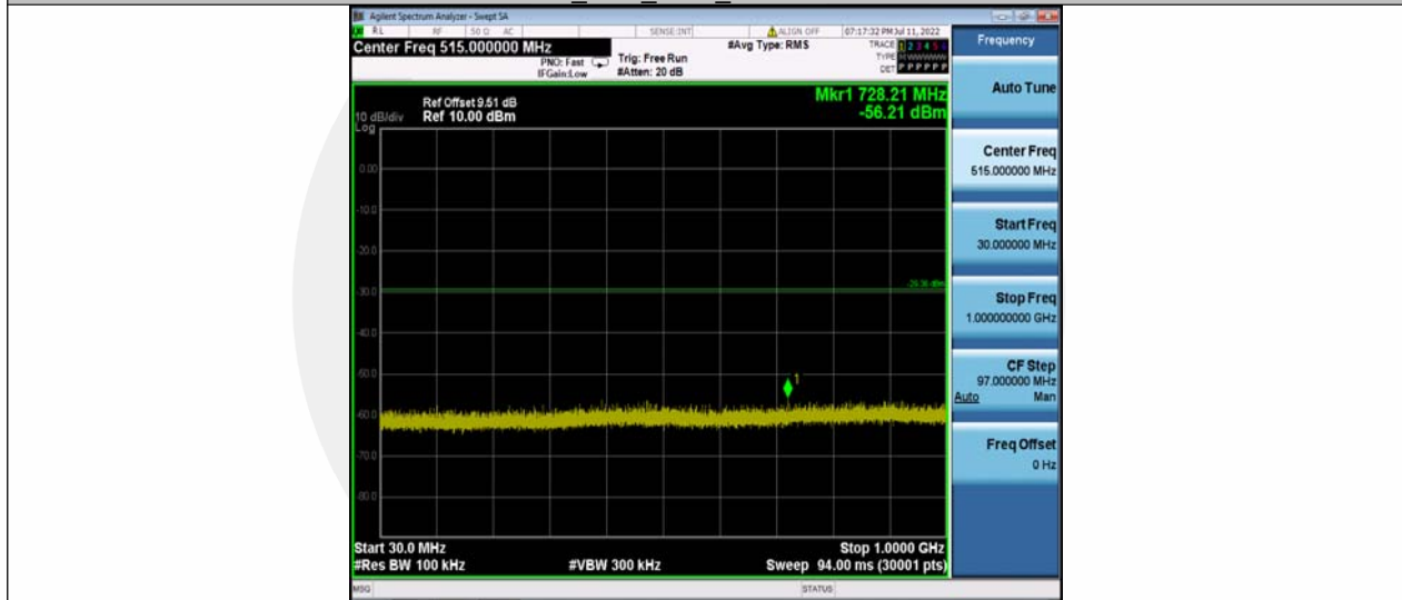
11B_Ant1_2412_30~1000
