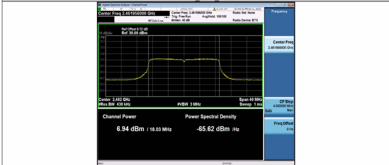
11N20SISO_Ant1_2462
