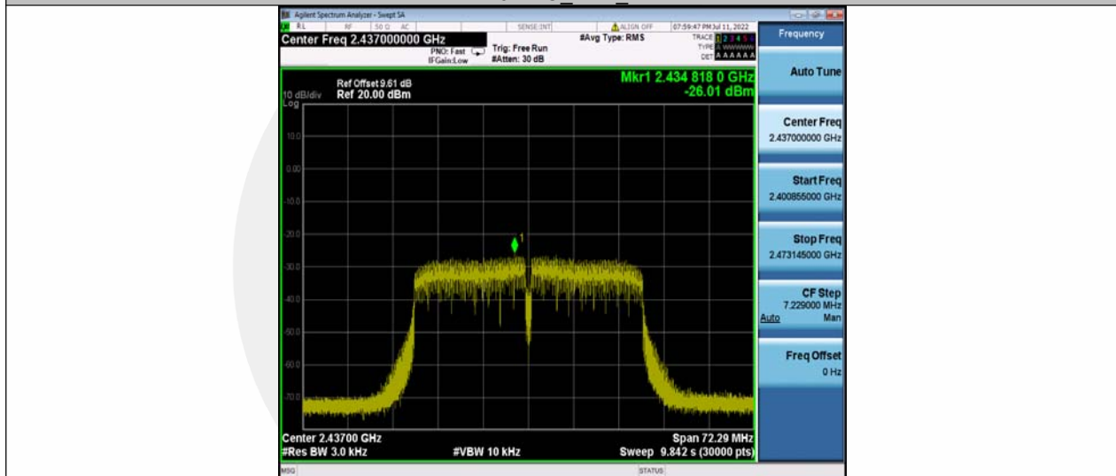
11N40SISO_Ant1_2437
