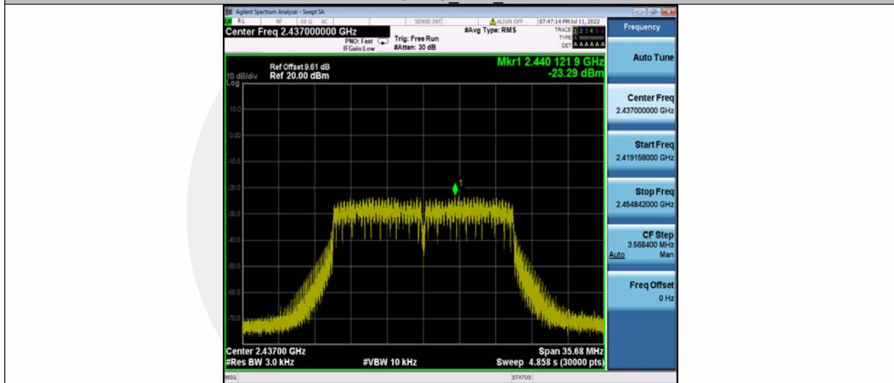
11N20SISO_Ant1_2437
