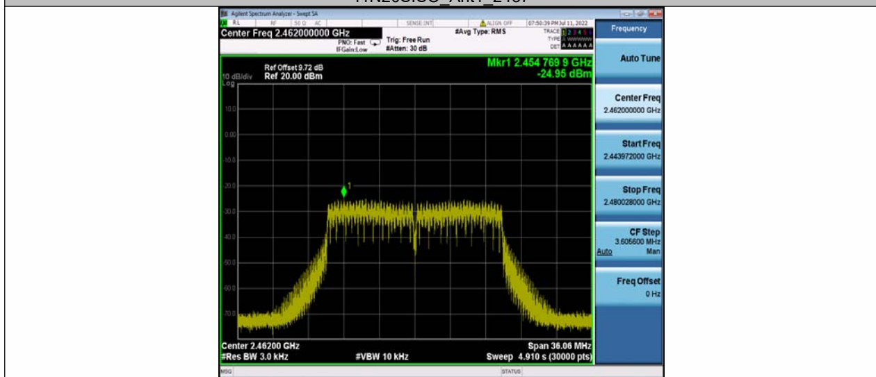
11N20SISO_Ant1_2462
