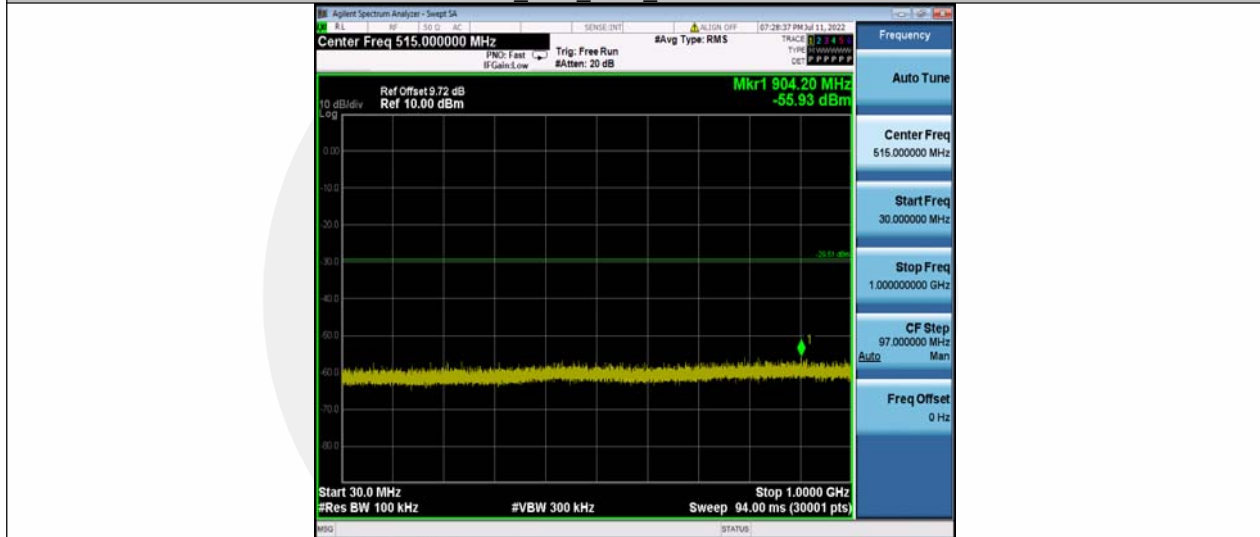
11B_Ant1_2462_30~1000
