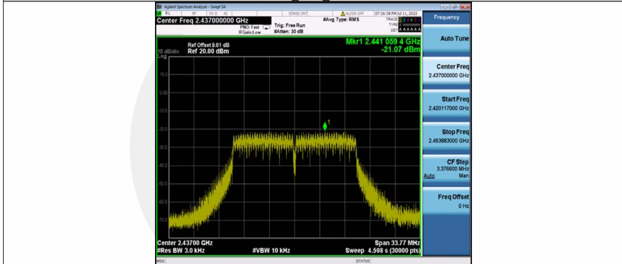
11G_Ant1_2437
