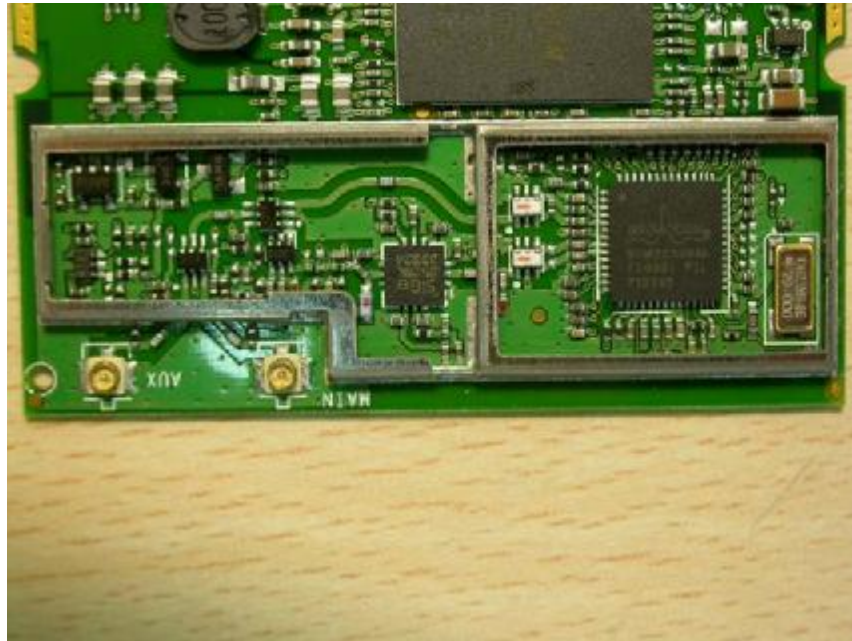
RF Module 4
