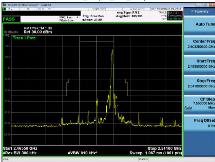
Band 41_16QAM_15M_RB1,74
