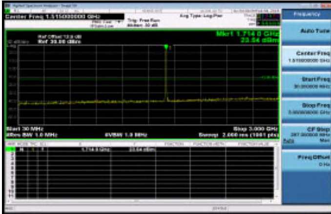
30MHz~3GHz_WCDMA_B4_LowCH1312-1712.4
