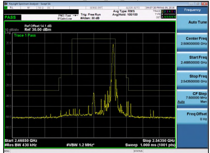
Band 41_QPSK_20M_RB1,99
