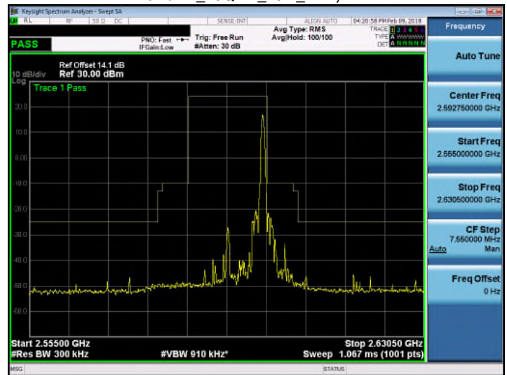
Band 41_16QAM_15M_RB1,74
