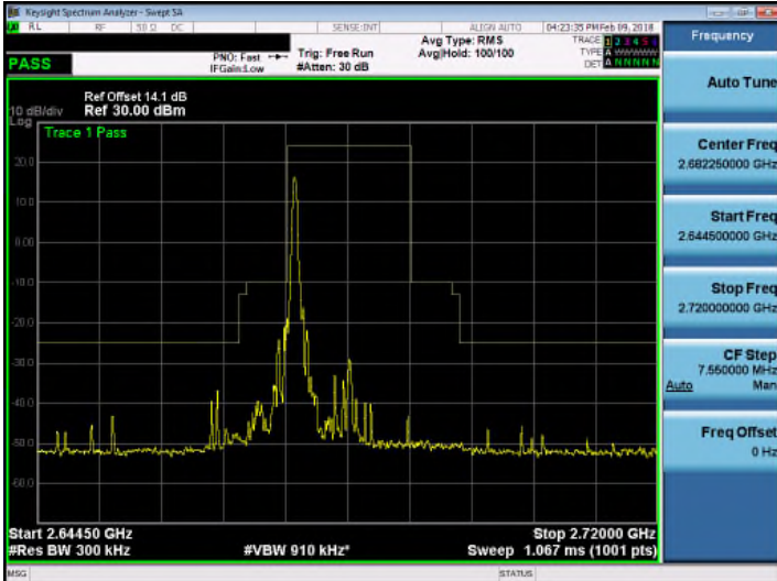
Band 41_16QAM_15M_RB1,74
