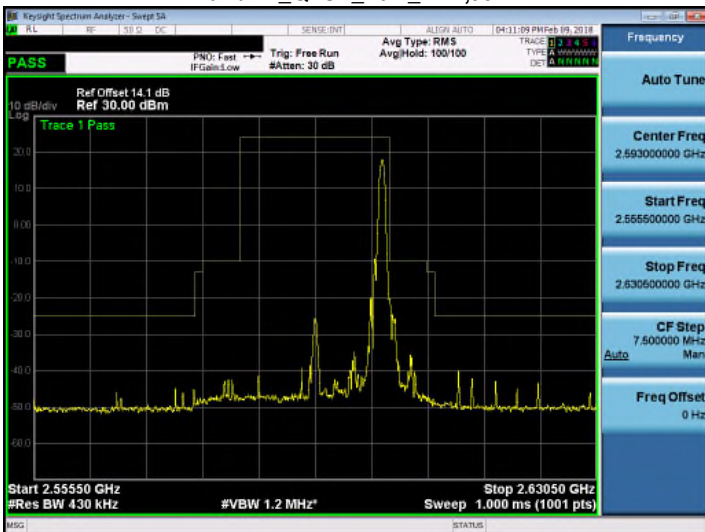
Band 41_QPSK_20M_RB1,99
