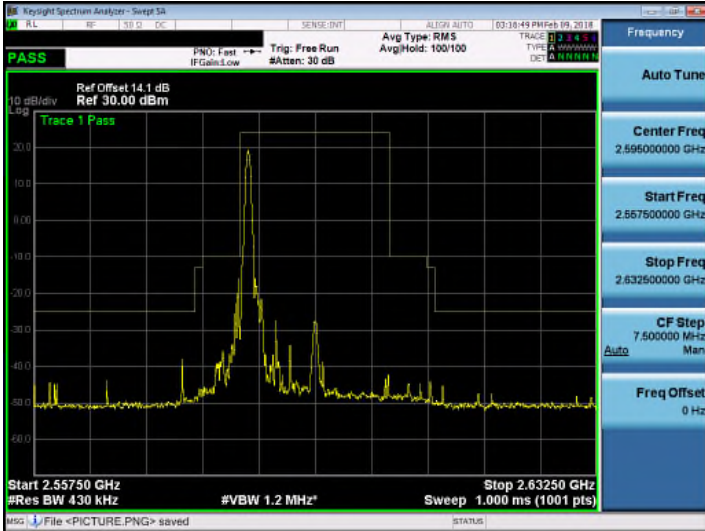
Band 38_QPSK_20M_RB1,99
