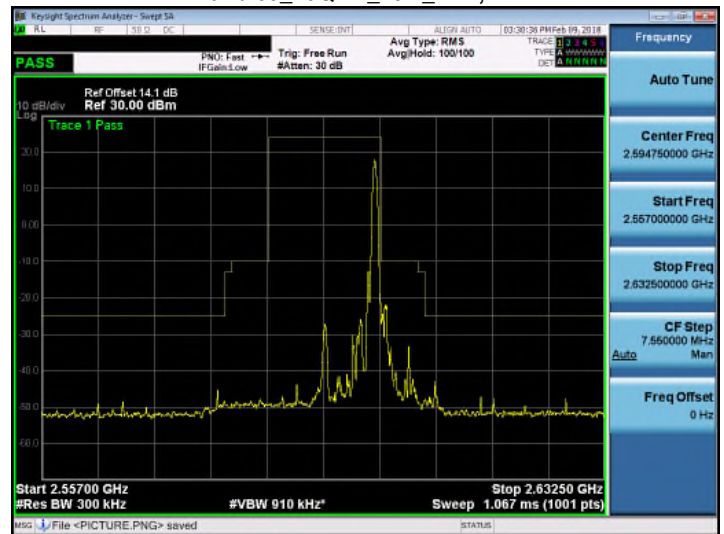
Band 38_16QAM_15M_RB1,74
