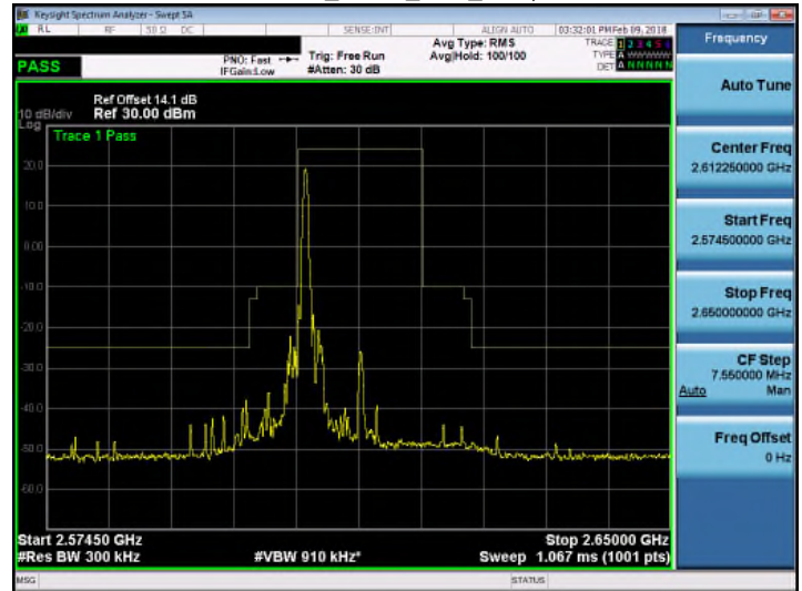
Band 38_QPSK_15M_RB1,74
