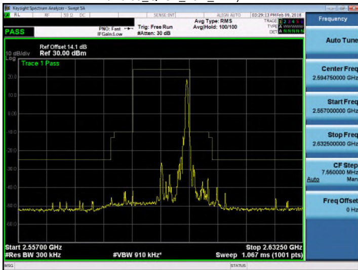
Band 38_QPSK_15M_RB1,74
