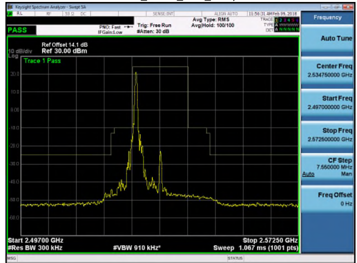
Band 7_QPSK_15M_RB1,74
