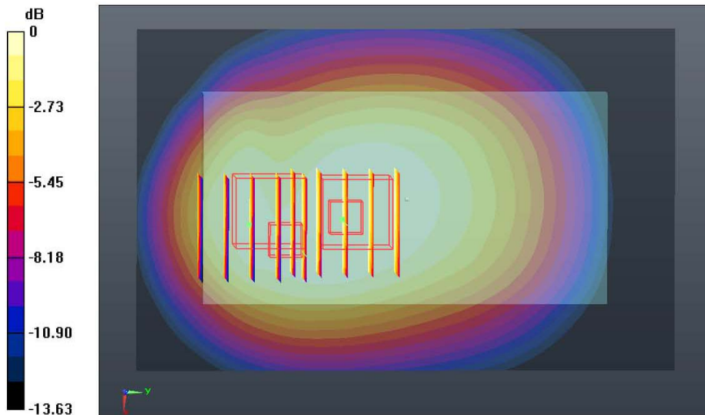
0 dB = 1.220mW/g
