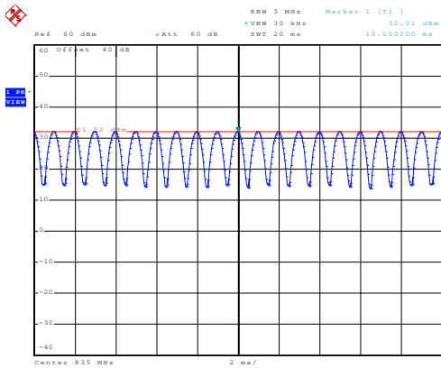
835MHz - CW
