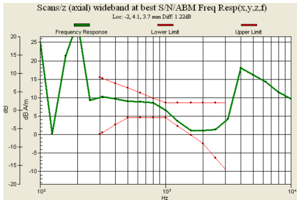
Fig. 9.1 GSM850 Ch128
