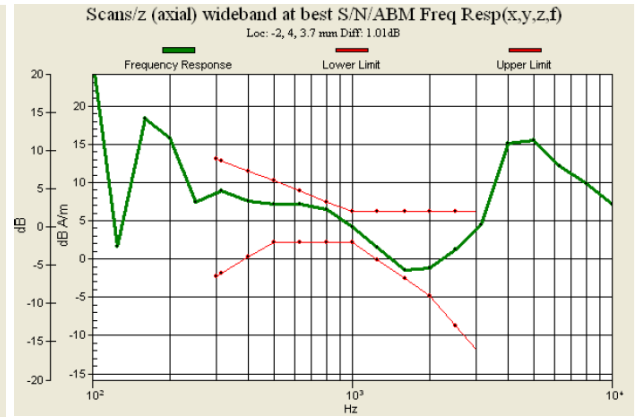
Fig. 9.2 WCDMA Band V Ch4182
