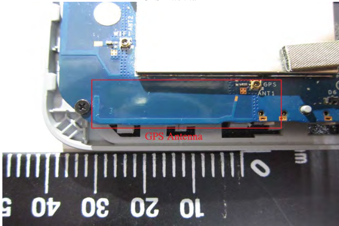
GPS Antenna
