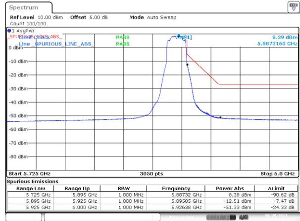
BE-NR-HIGH, MIMO-A, 802.11n20-HT8, Ch177
