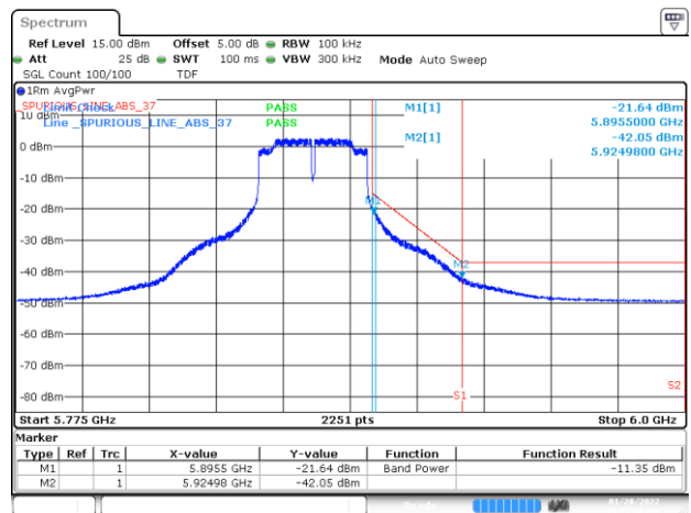
BE-NR-HIGH, SISO-A, 802.11n40-HT0, Ch175
