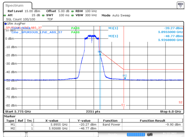
BE-NR-HIGH, SISO-A, 802.11n20-HT0, Ch177
