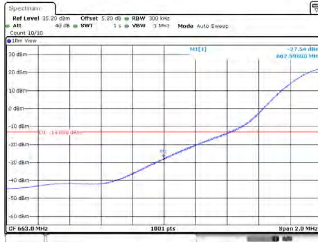
Band71_20MHz_QPSK_133222_100RB#0
