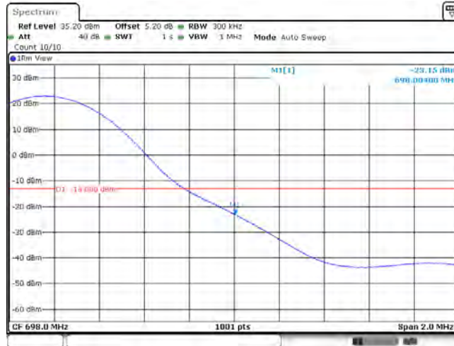
Band71_15MHz_QPSK_133397_75RB#0
