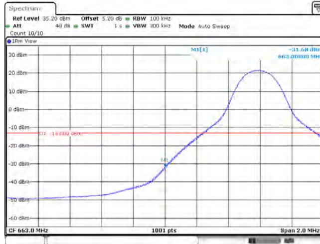
Band71_10MHz_QPSK_133172_50RB#0
