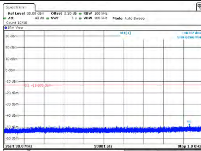
Band66_20MHz_QPSK_132072_1RB#0
