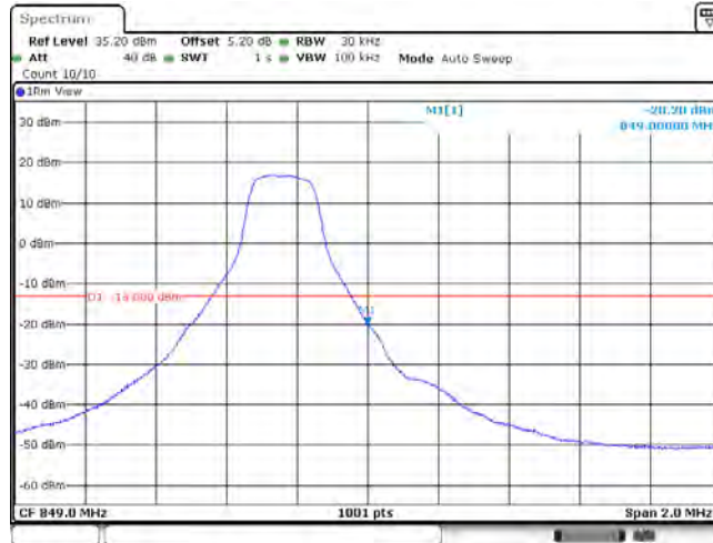
Band5_3MHz_QPSK_20635_15RB#0
