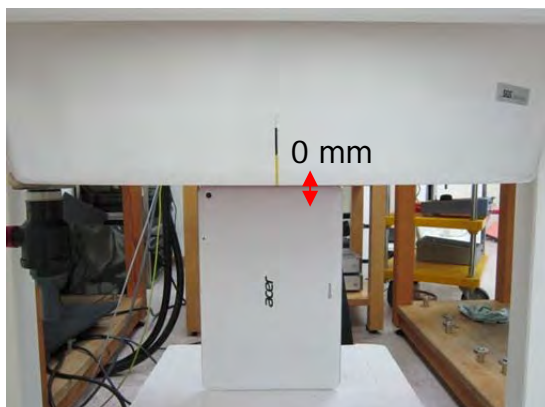
Fig.4 EUT Left edge to flat phantom
