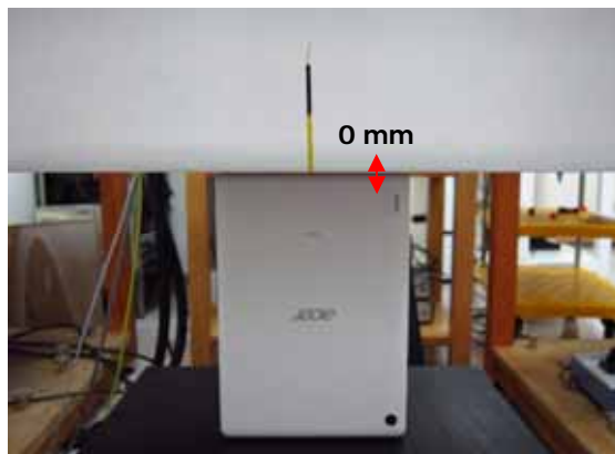
Fig.5 EUT Edge 3 to flat phantom
