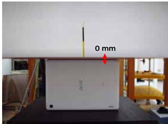
Fig.4 EUT Edge 1 to flat phantom
