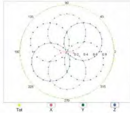
f=1800 MHz,R22
