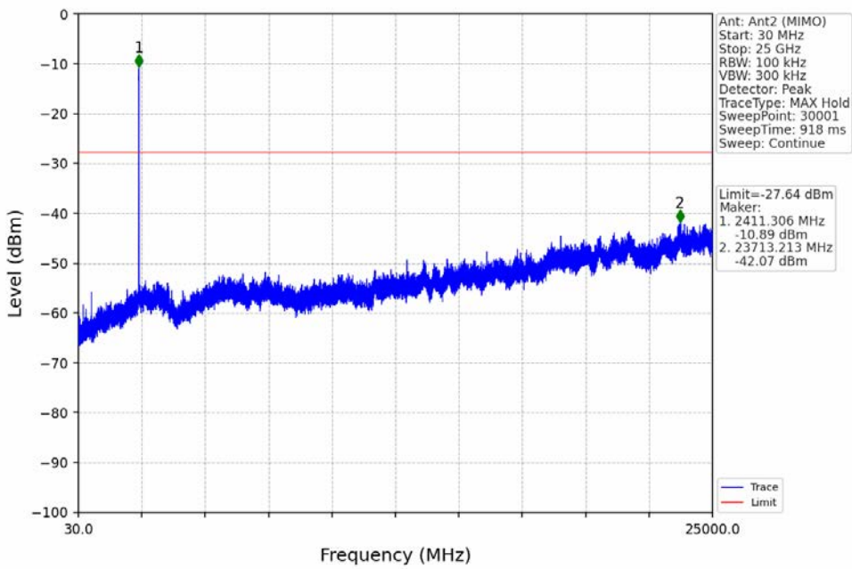
802.11n(HT20)_LCH_2412MHz_Ant2 (MIMO)_NTNV
