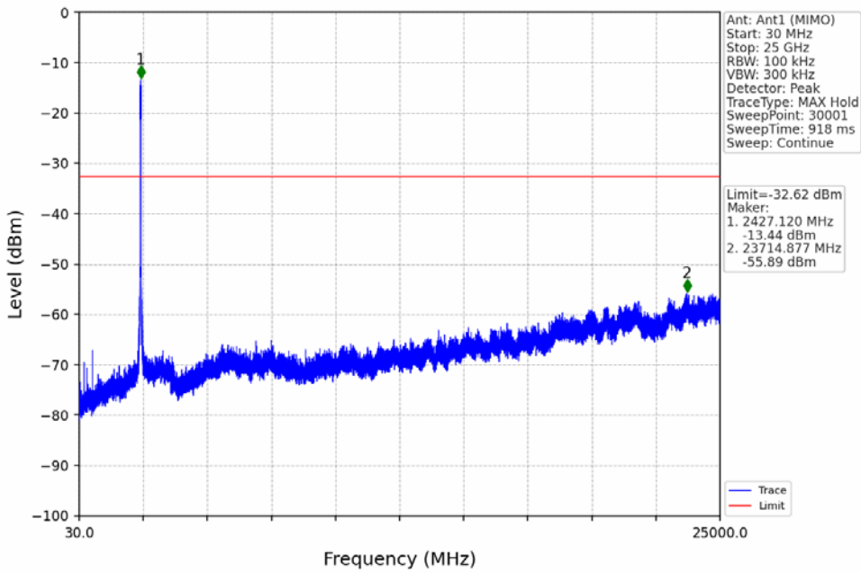
802.11ax(HEW40)_LCH_2422MHz_RU484_Left_Ant1 (MIMO)_NTNW
