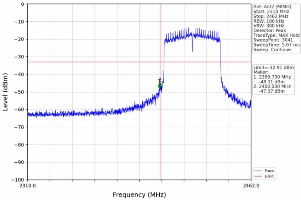
802.11ax(HEW40)_LCH_2422MHz_RU484_Left_Ant2 (MIMO)_NTNW
