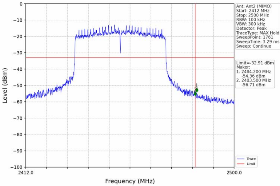
802.11ax(HEW40)_HCH_2452MHz_RU484_Left_Ant2 (MIMO)_NTNV
