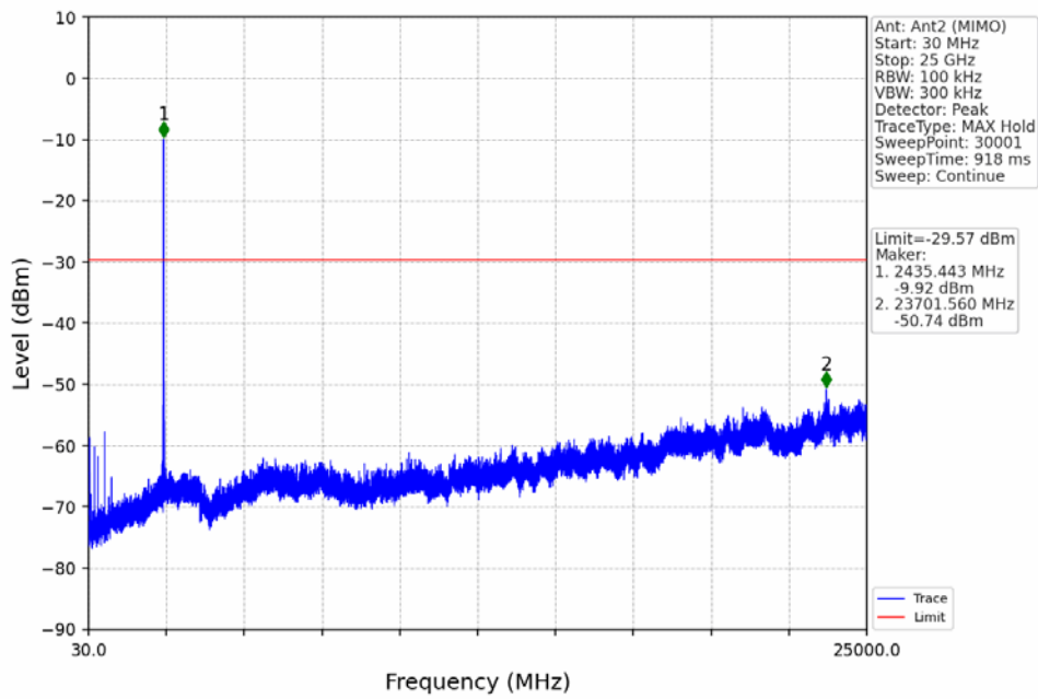
802.11ax(HEW20)_MCH_2437MHz_RU242_Left_Ant2 (MIMO)_NTNV
