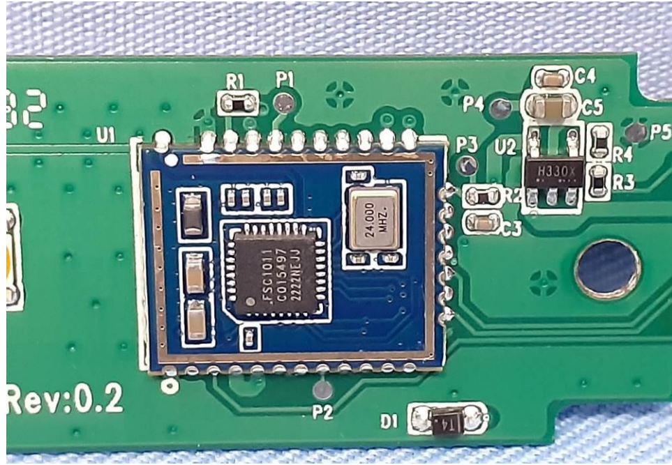
EUT Photo (21)
