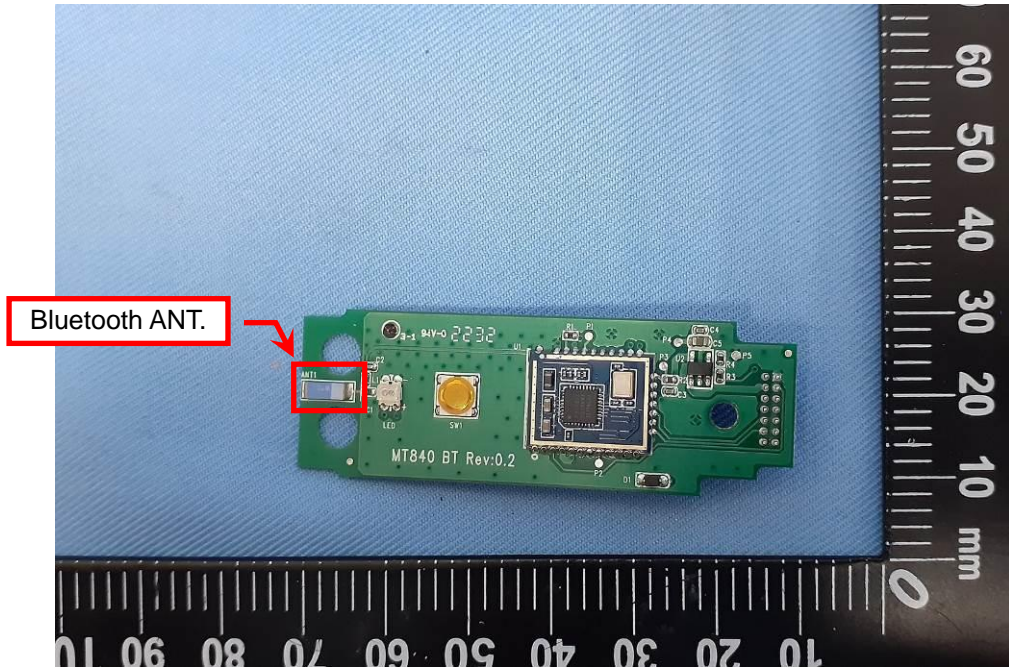
EUT Photo (20)
