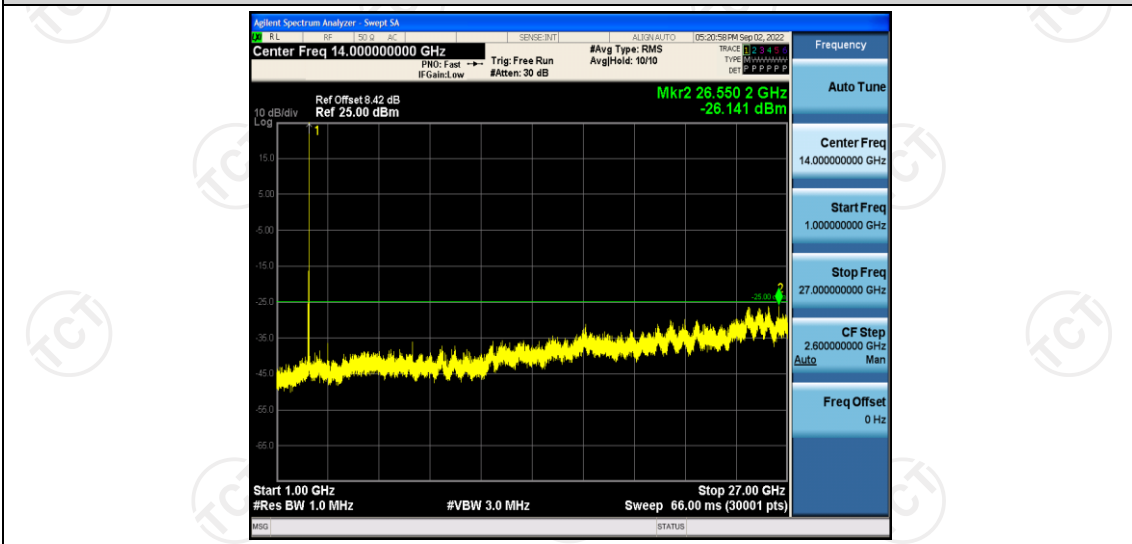
Band41-20MHz-16QAM-41140-1RB#0-Range2:1000~27000MHz
