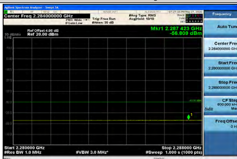
Band40-5MHz-QPSK-39225-1RB#24-Range1:2280~2288MHz
