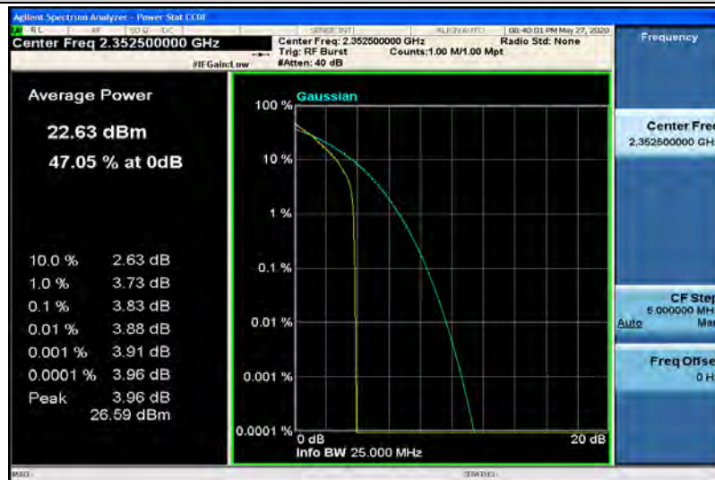
Band40-5MHz-QPSK-39200-1RB#0
