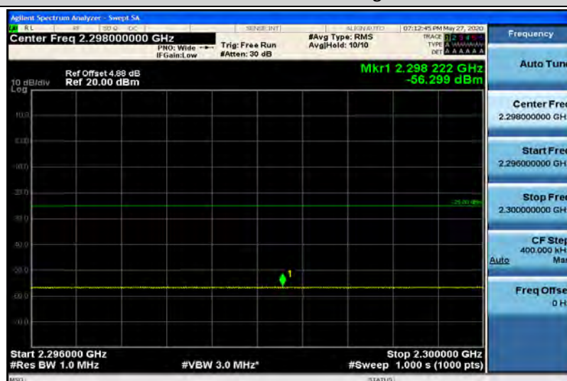
Band40-5MHz-QPSK-39200-1RB#0-Range4:2296~2300MHz
