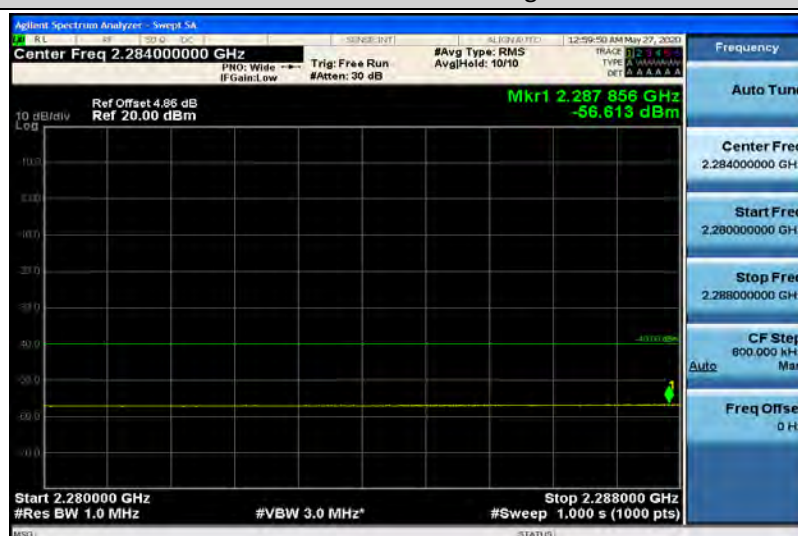
Band40-5MHz-QPSK-38775-1RB#0-Range1:2280~2288MHz
