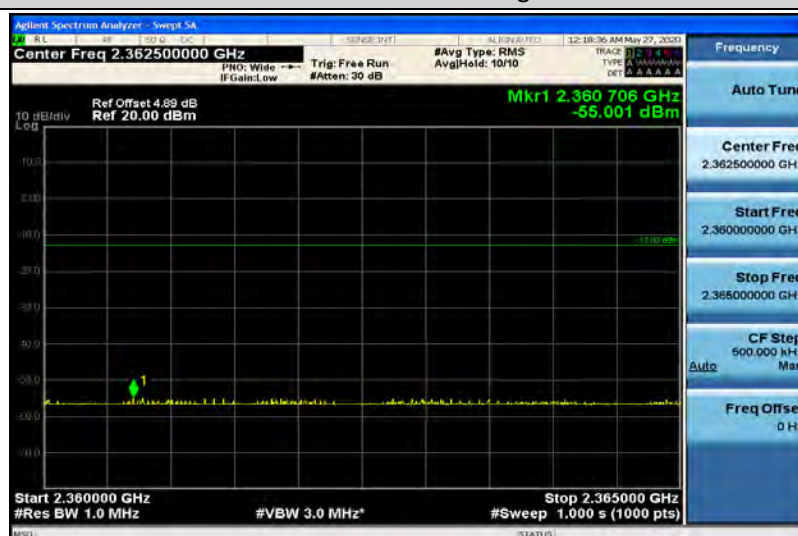
Band40-5MHz-QPSK-38725-1RB#0-Range13:2360~2365MHz
