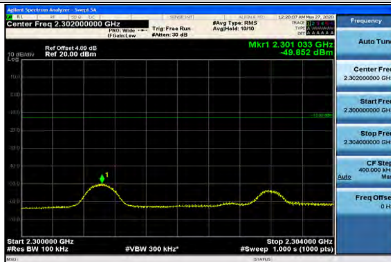
Band40-5MHz-16QAM-38725-1RB#0-Range5:2300~2304MHz
