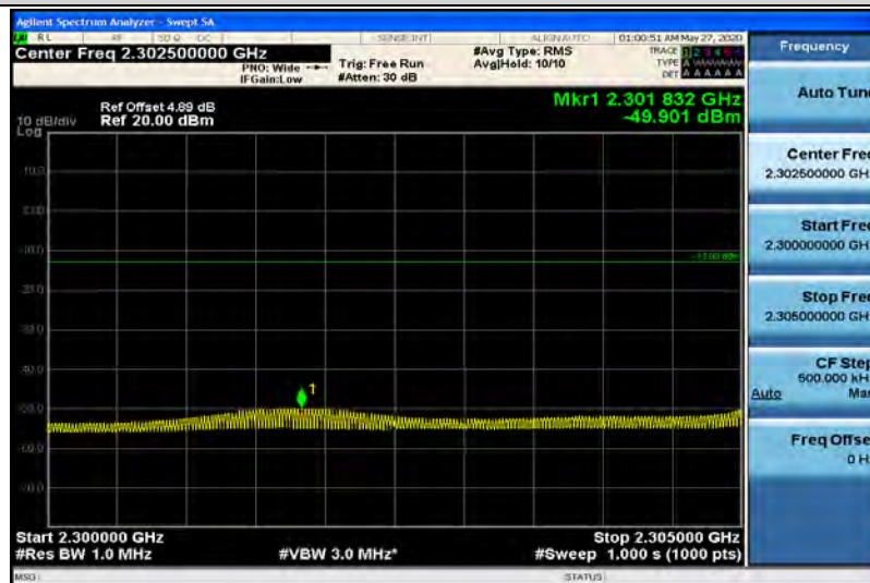
Band40-5MHz-QPSK-38775-1RB#0-Range5:2300~2305MHz
