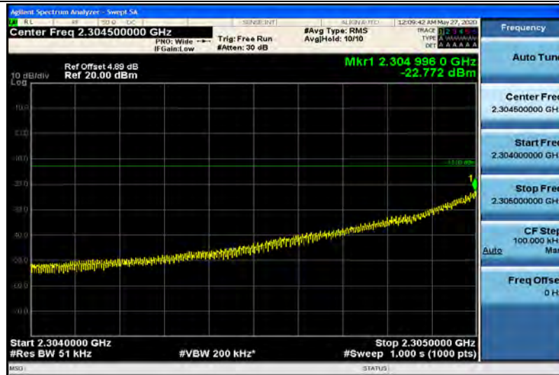
Band40-5MHz-QPSK-38725-1RB#24-Range6:2304~2305MHz
