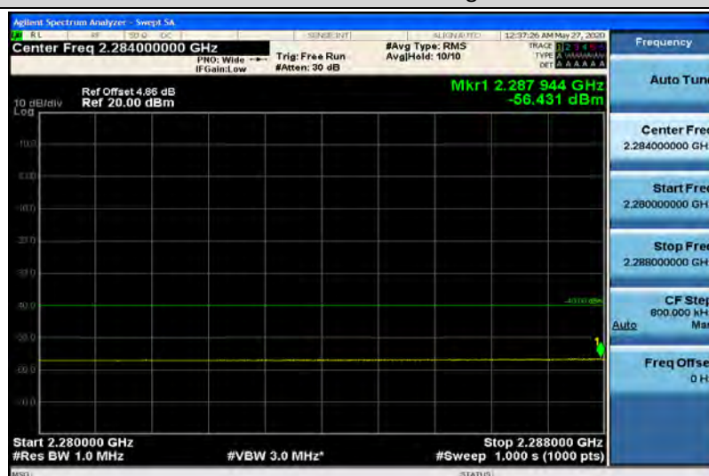
Band40-5MHz-QPSK-38750-1RB#0-Range1:2280~2288MHz
