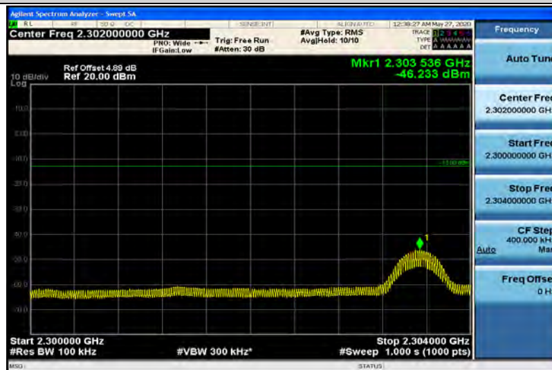
Band40-5MHz-QPSK-38750-1RB#0-Range5:2300~2304MHz
