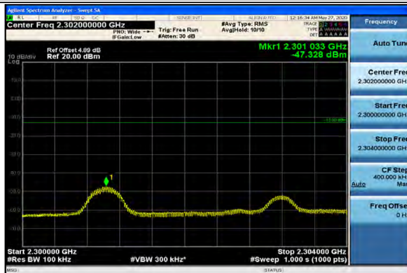
Band40-5MHz-QPSK-38725-1RB#0-Range5:2300~2304MHz
