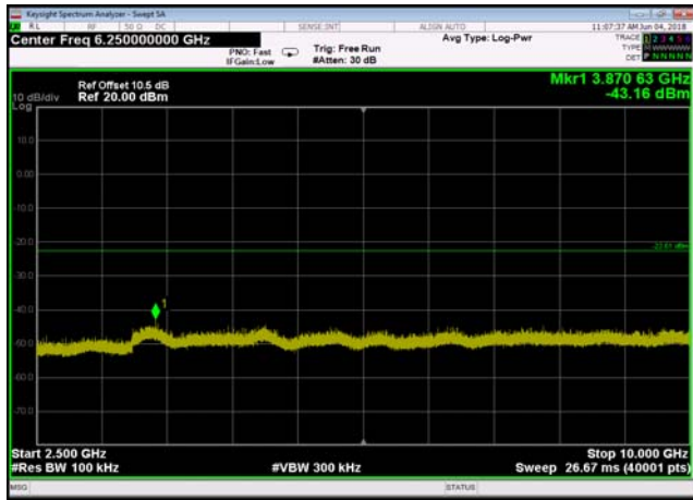
,Plot 4,2500MHz~10000MHz-802.11n(HT40),2452MHz,
