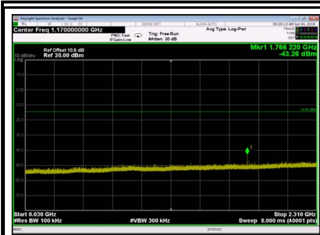
,Plot 3,30MHz~2310MHz-802.11b,2462MHz
