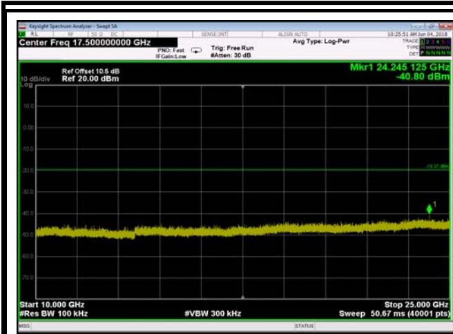
,Plot 5,10000MHz~25000MHz-802.11n(HT20),2462MHz,
