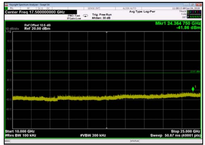
,Plot 5,10000MHz~25000MHz-802.11n(HT40),2452MHz,
