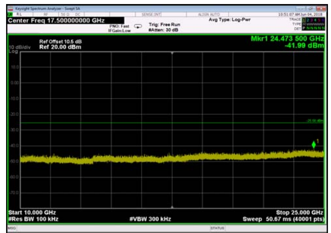
,Plot 5,10000MHz~25000MHz-802.11n(HT40),2452MHz,
