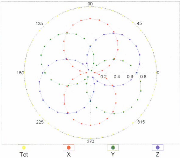
f=450 MHz,TEM
