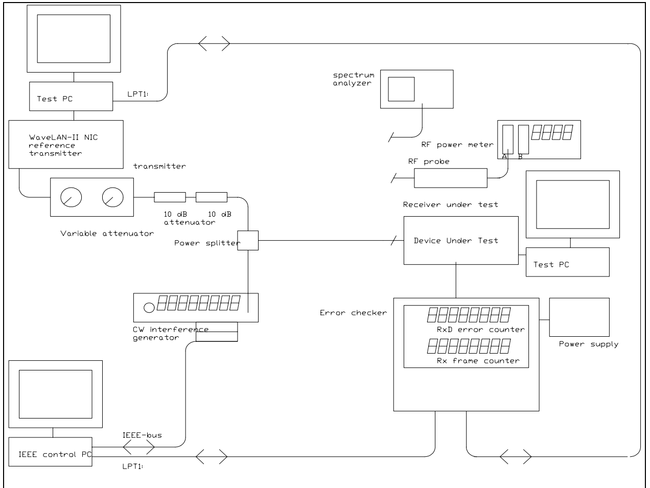
Fig. 1 Test Setup
