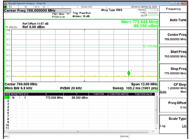
Band13_10MHz_QPSK_RB50_0_CH23230
