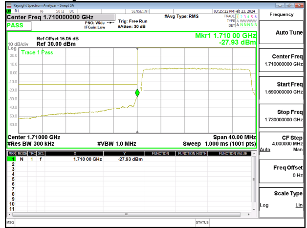
Band Edge_Band4_20MHz_QPSK_RB100_0_CH20300
