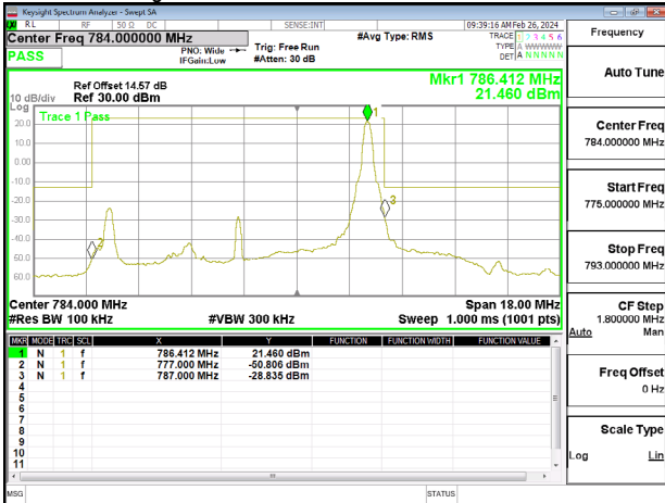
Band Edge_Band13_10MHz_QPSK_RB50_0_CH23230
