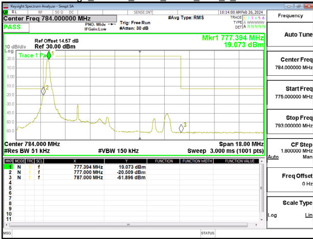
Band Edge_Band13_5MHz_QPSK_RB1_24_CH23255
