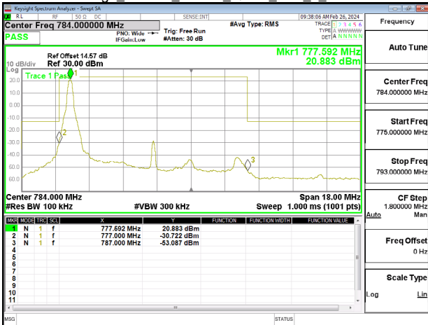
Band Edge_Band13_10MHz_QPSK_RB1_49_CH23230
