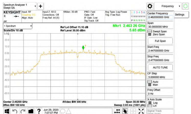
FCC_15_247_WLAN\Reference Level_802.11g_20MHz_Chain0_2462MHz
