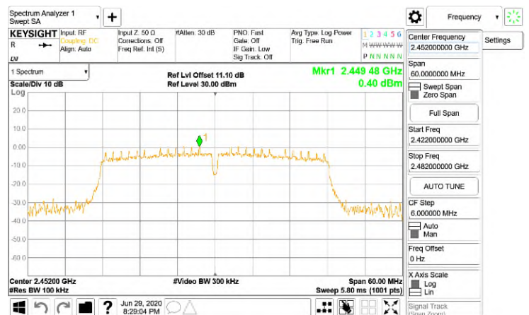
FCC_15_247_WLAN\Reference Level_802.11n_40MHz_Chain0_2452MHz
