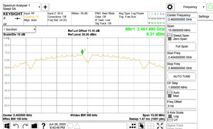
FCC_15_247_WLAN\Reference Level_802.11b_20MHz_Chain0_2462MHz
