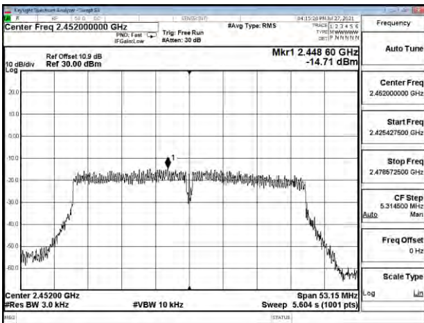
802.11ac_40MHz_Chain0_2452MHz
