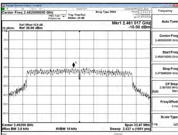
802.11ac_20MHz_Chain0_2462MHz
