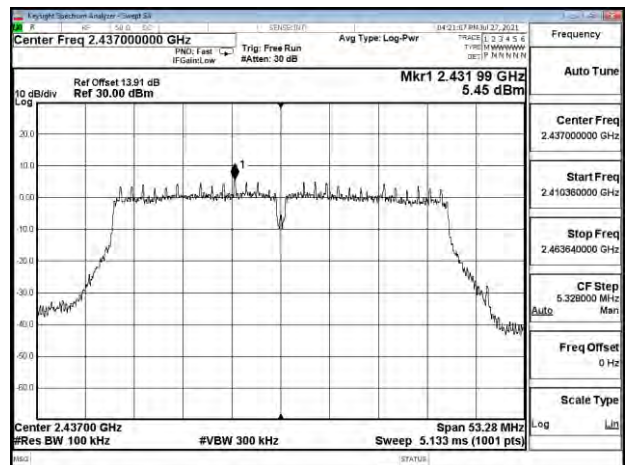
802.11ac_40MHz_Chain0_2437MHz
