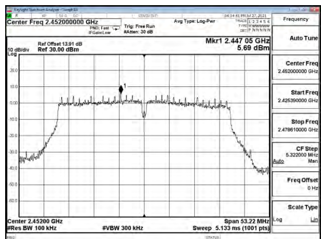
802.11ac_40MHz_Chain0_2452MHz
