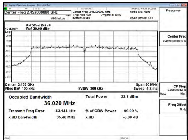
802.11ac_40MHz_Chain1_2452MHz
