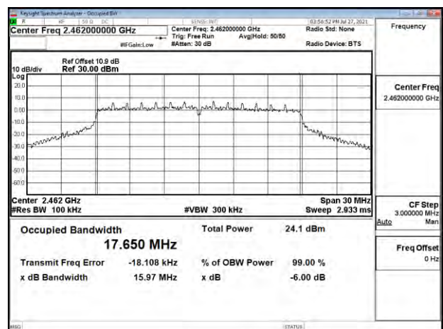
802.11ac_20MHz_Chain1_2462MHz
