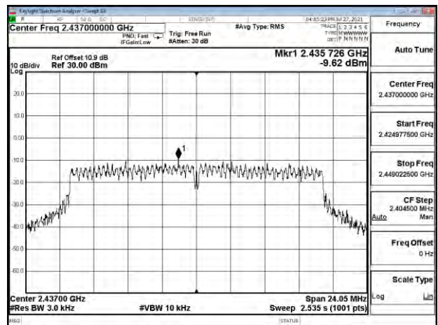
802.11ac_20MHz_Chain1_2437MHz
