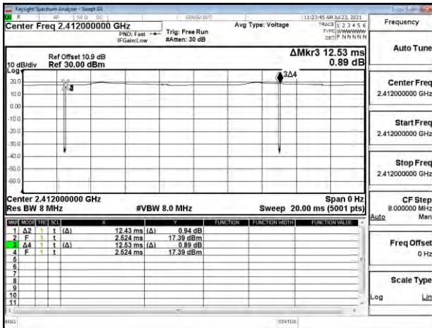
802.11b_20MHz_Chain0_2412MHz
