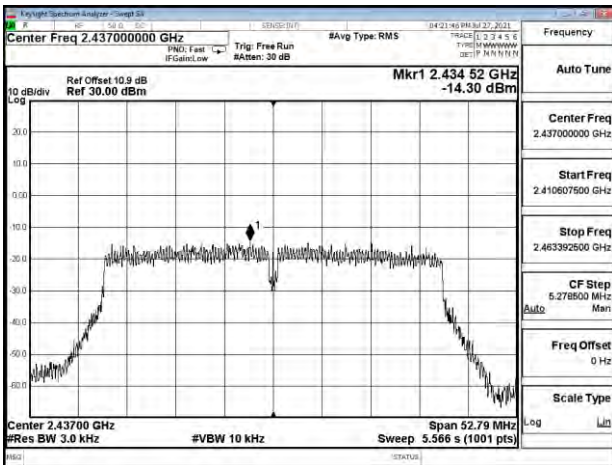
802.11ac_40MHz_Chain0_2437MHz
