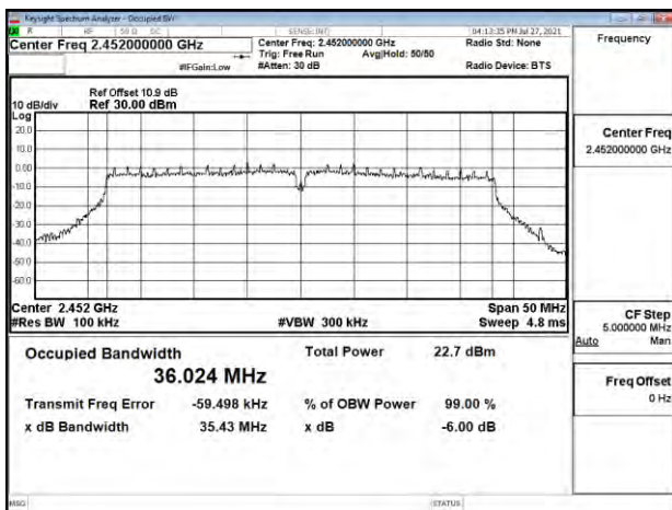
802.11ac_40MHz_Chain0_2452MHz
