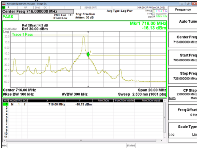
Band Edge\Band12_10MHz\QPSK_RB1_49_CH23130
