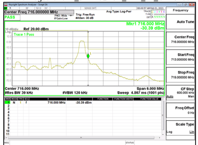
Band Edge\Band12_3MHz\QPSK_RB1_14_CH23165
