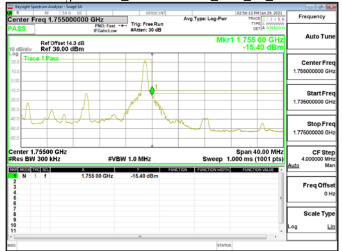
Band Edge\Band4_20MHz\QPSK_RB1_99_CH20300
