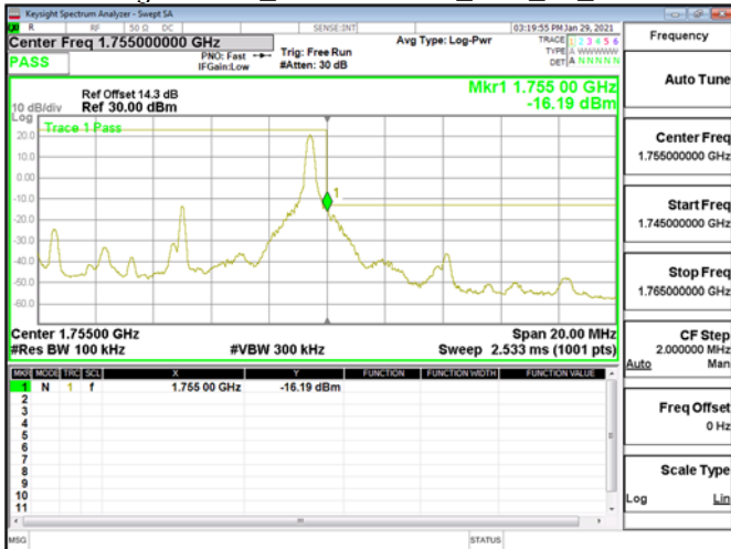
Band Edge\Band4_10MHz\QPSK_RB1_49_CH20350
