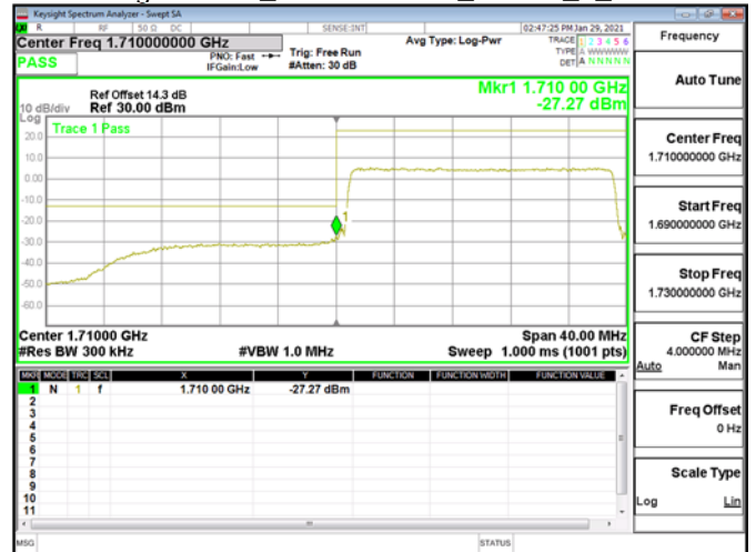
Band Edge\Band4_20MHz\QPSK_RB100_0_CH20050
