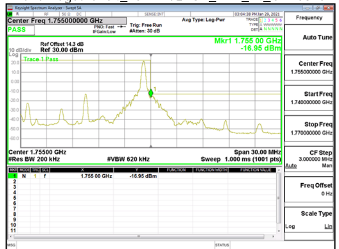
Band Edge\Band4_15MHz\QPSK_RB1_74_CH20325
