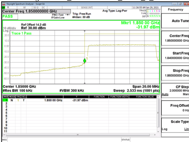
Band Edge\Band2_10MHz\QPSK_RB50_0_CH18650
