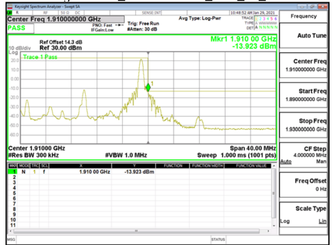
Band Edge\Band2_20MHz\QPSK_RB1_99_CH19100
