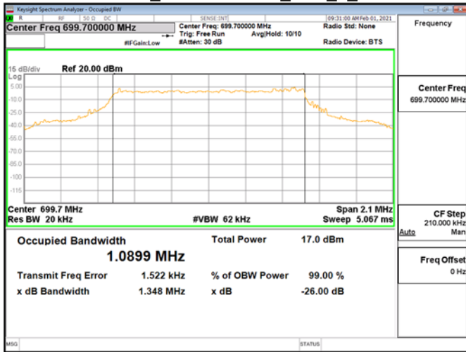
OBWBand12_1.4MHz\QPSK_RB6_0_CH23017
