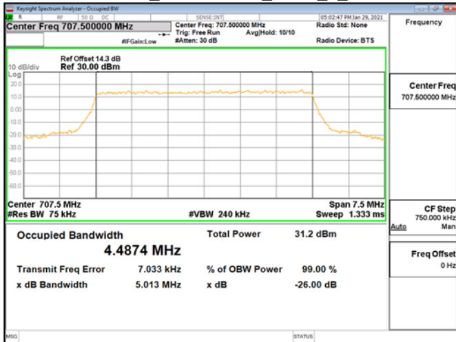
OBWBand12_5MHzQPSK_RB25_0_CH23095
