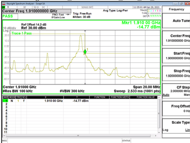
Band Edge\Band2_10MHz\QPSK_RB1_49_CH19150
