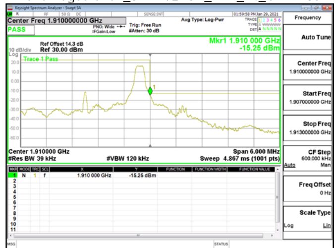
Band Edge\Band2_3MHz\QPSK_RB1_14_CH19185
