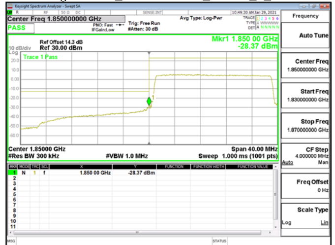
Band Edge\Band2_20MHz\QPSK_RB100_0_CH18700
