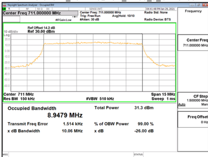
OBWBand12_10MHz\QPSK_RB50_0_CH23130
