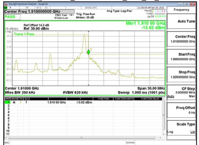
Band Edge\Band2_15MHz\QPSK_RB1_74_CH19125
