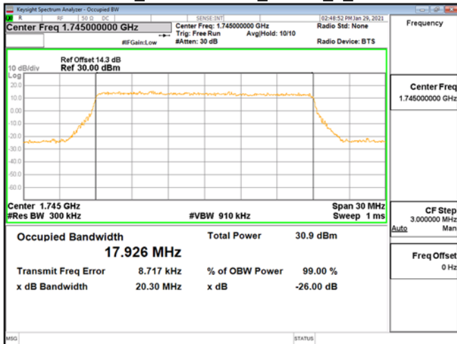
OBWBand4_20MHz\QPSK_RB100_0_CH20300
