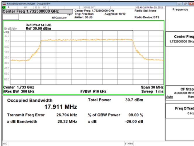
OBWBand4_20MHz\QPSK_RB100_0_CH20175
