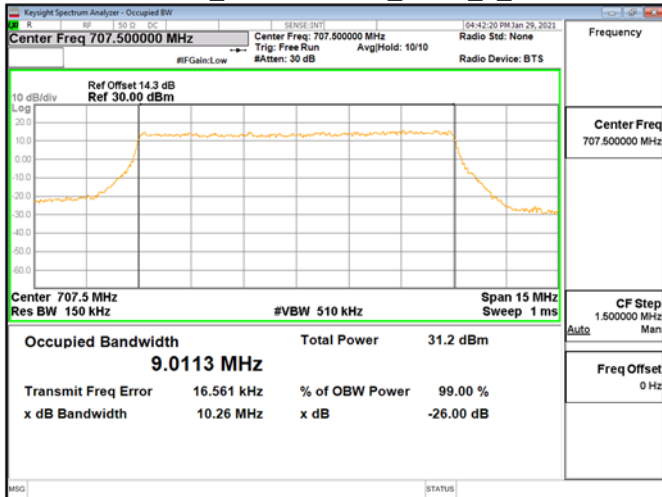
OBWBand12_10MHz\QPSK_RB50_0_CH23095
