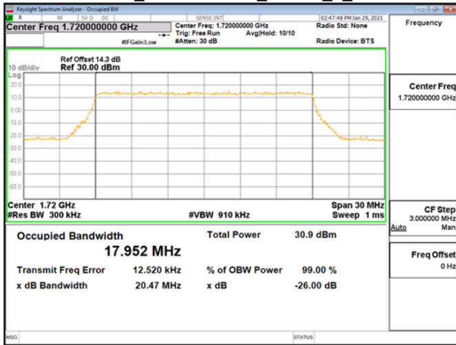
OBWBand4_20MHz\QPSK_RB100_0_CH20050
