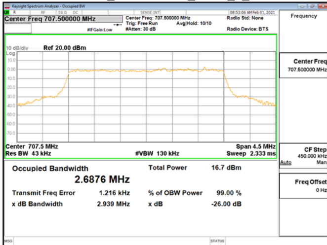
OBWBand12_3MHzQPSK_RB15_0_CH23095
