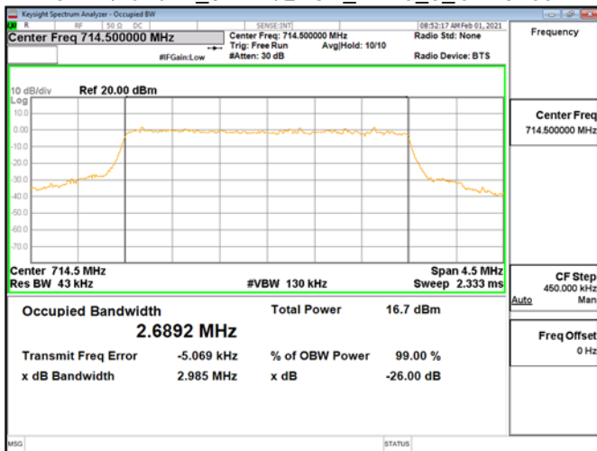
OBWBand12_3MHzQPSK_RB15_0_CH23165
