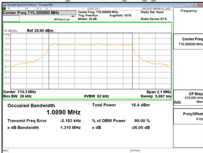
OBWBand12_1.4MHz\QPSK_RB6_0_CH23173
