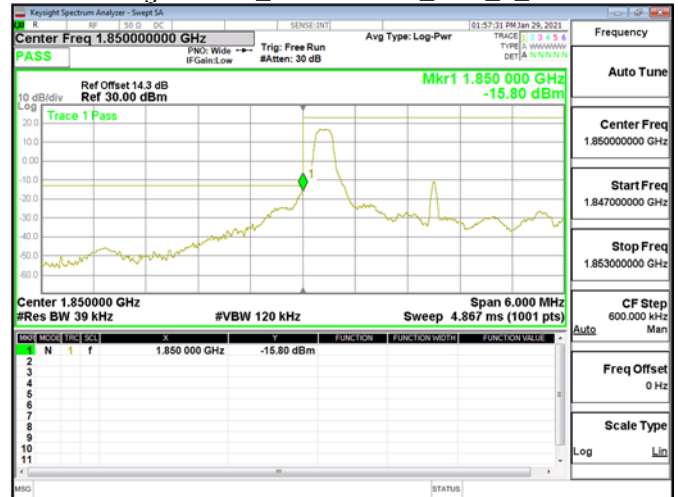
Band Edge\Band2_3MHz\QPSK_RB1_0_CH18615
