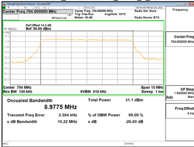
OBWBand12_10MHz\QPSK_RB50_0_CH23060
