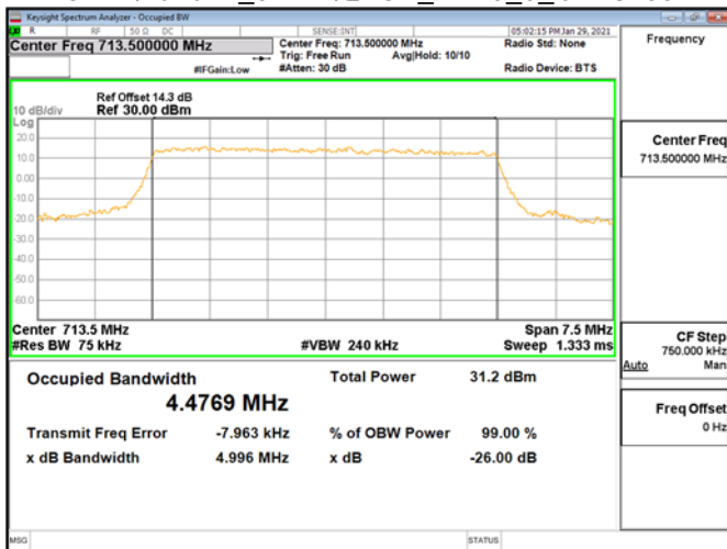
OBWBand12_5MHzQPSK_RB25_0_CH23155
