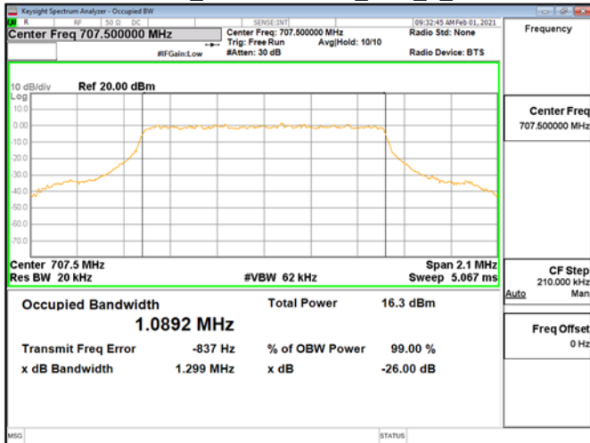
OBWBand12_1.4MHz\QPSK_RB6_0_CH23095
